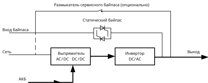
Рисунок 2.5. Функциональная схема ИБП при работе от АКБ
