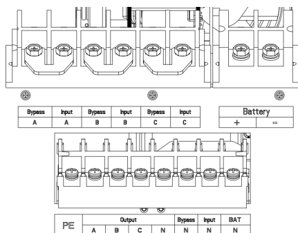
(б) Силовые клеммы ИБП мощностью 30-40 кВА с отсеком для встроенных АКБ Рисунок 3.7. Силовые клеммы
