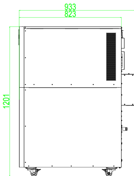
(б) 30; 40 кВА с отсеком для встроенных АКБ (ед. изм.: мм)
