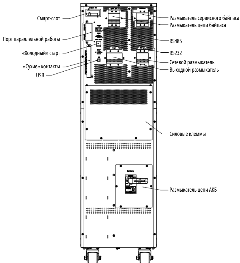
(в) ИБП мощностью 30-40 кВА с отсеком для встроенных АКБ, вид сзади
