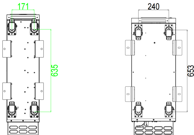
ИБП 10-20 кВА и 30-40 кВА с отсеком для встроенных АКБ (вид снизу, ед. изм.: мм)
